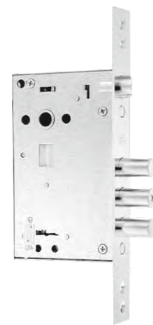
1 Крит-30 4Л основной замок сувальдного типа 2 класс взломостойкости количество ригелей 3 диаметр ригелей 16 мм вылет ригелей 21 мм количество оборотов 3
